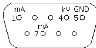
Рис.1. Цоколевка информационного разъема DB-9M
